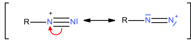
Abb. 13: Mesomere Grenzstrukturen der Diazoniumgruppe.
