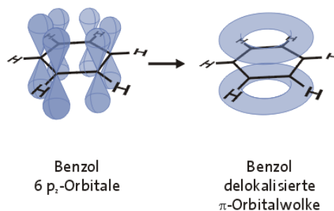
Abb. 7: [5] Delokalisierung der \pi -Elektronen im Benzolmolekül
