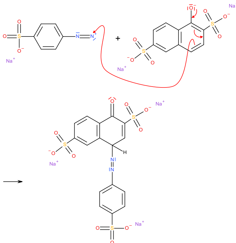
Abb. 14: Azokupplung.
